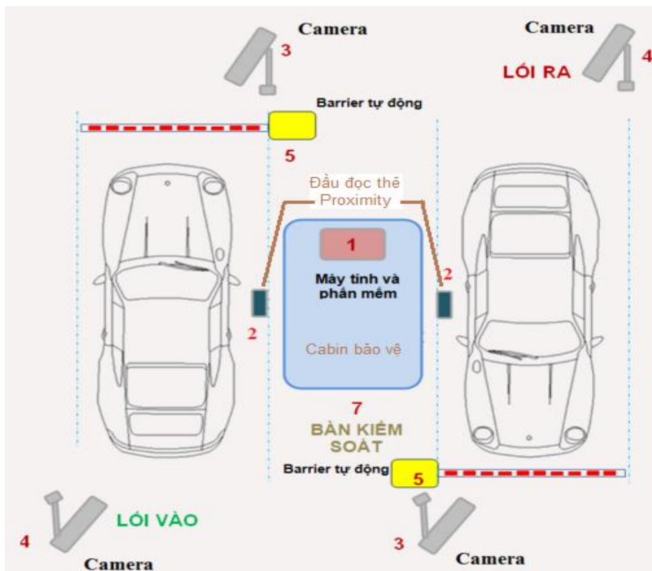
Sơ đồ hệ thống kiểm soát bãi đậu xe một lối vào một lối ra
