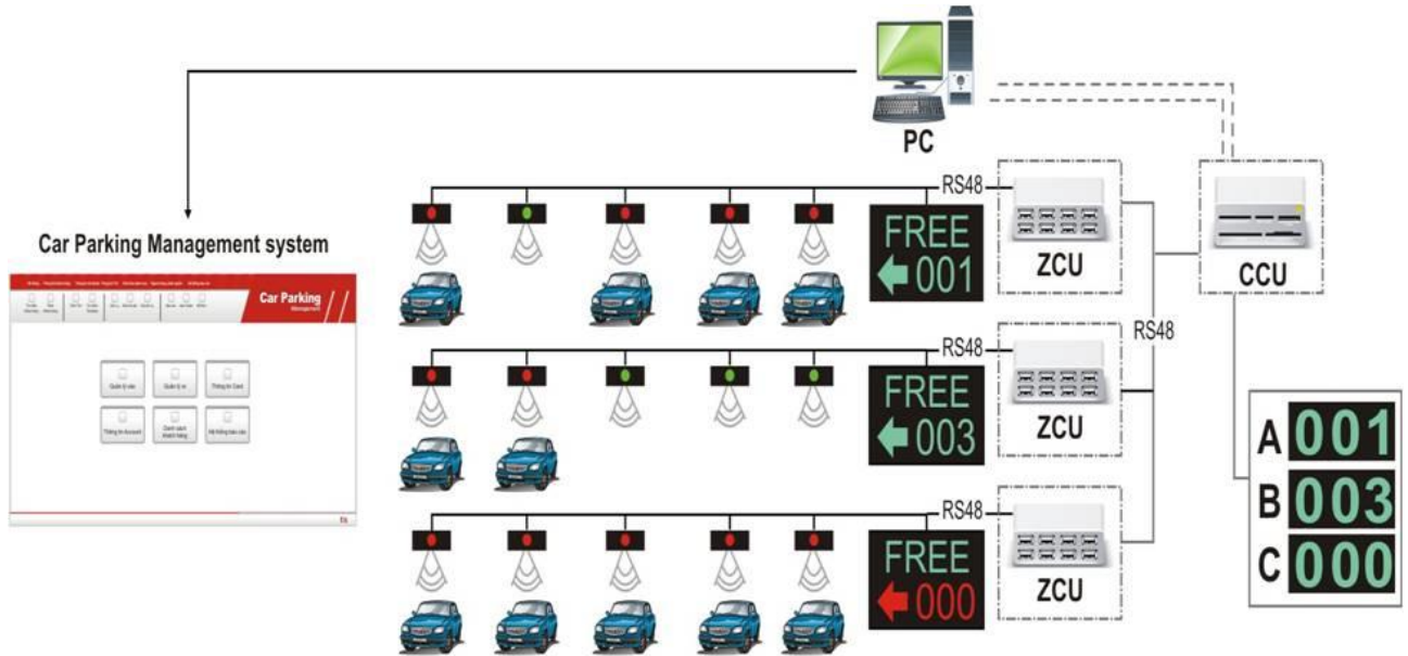
Sơ đồ điều khiển và quản lý hệ thống bãi đậu xe
